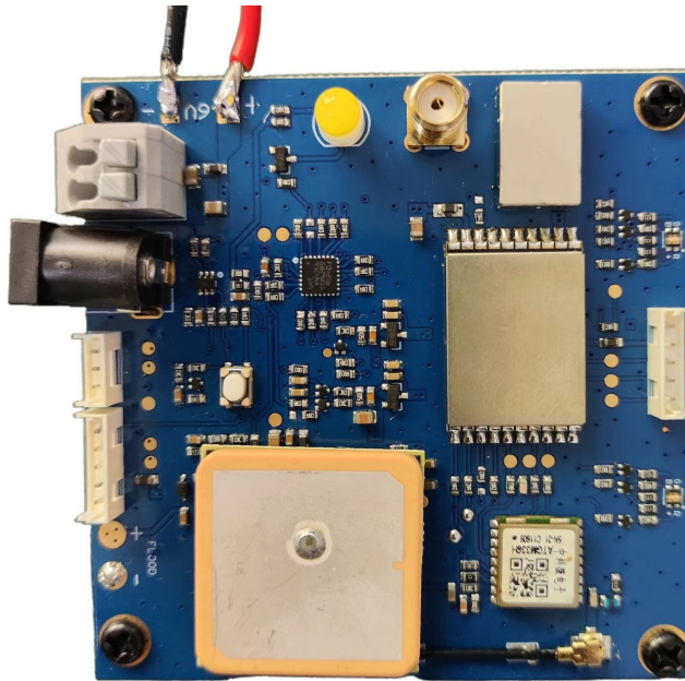
图六 评估板(实物拍照)
