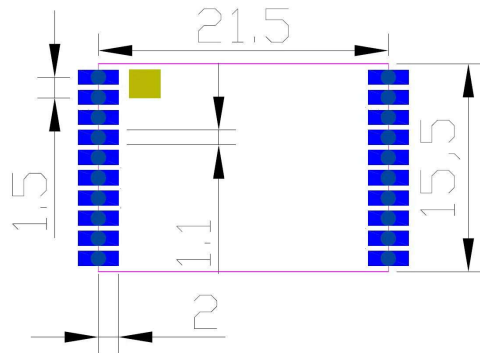
图二 模组尺寸 (21.5mm*15.5mm*3.5mm)
