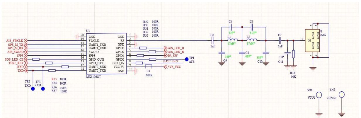
图四 应用电路示例
