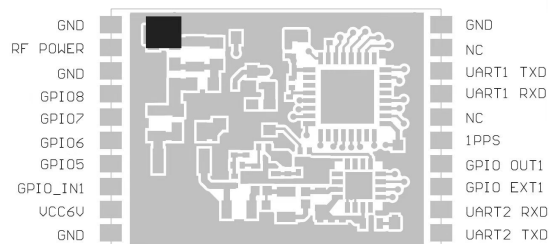
图三 模组管脚分布
