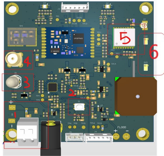
图五 评估板示意图
